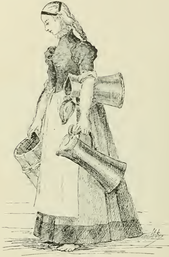
Fig. 327. — Servante Allemande.
